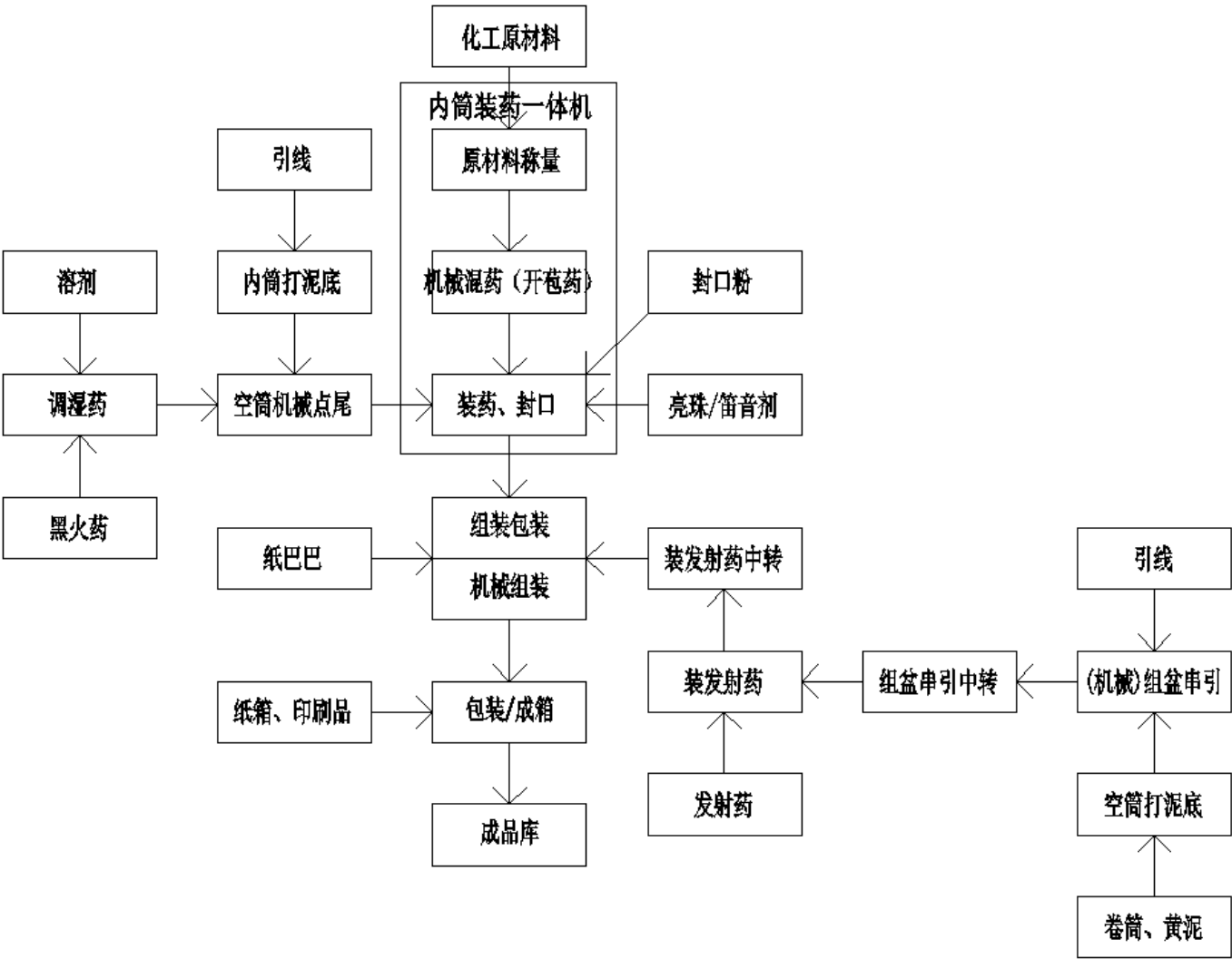
图 2-1 C 级组合烟花类产品生产工艺流程图
