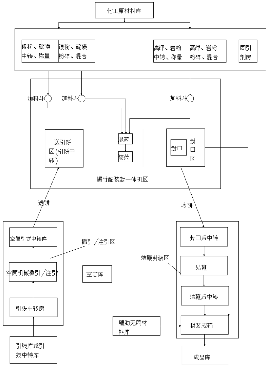
图 2-4 C 级爆竹类产品生产工艺流程图
