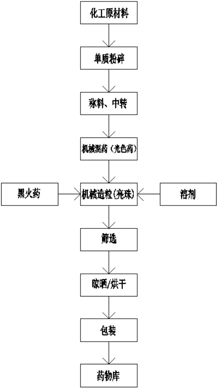
图 2-5 烟火药（亮珠）生产工艺流程图
