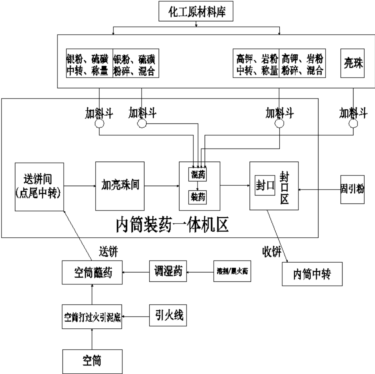
图 2-2 组合烟花内筒装药一体机生产工艺流程图
